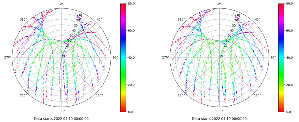
Skyplot for station VIGO. Parameter M1C Data file VIGO00ESP_R_2022109.xtr Skyplot for station VIGO. Parameter M2C Data file VIGO00ESP_R_2022109.xtr
