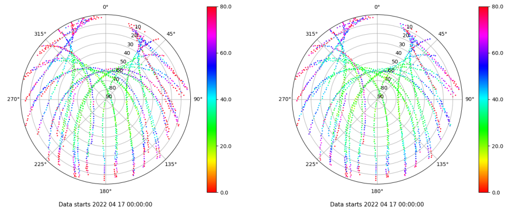
Skyplot for station VIGO. Parameter M1C Data file VIGO00ESP_R_2022107.xtr Skyplot for station VIGO. Parameter M2C Data file VIGO00ESP_R_2022107.xtr
