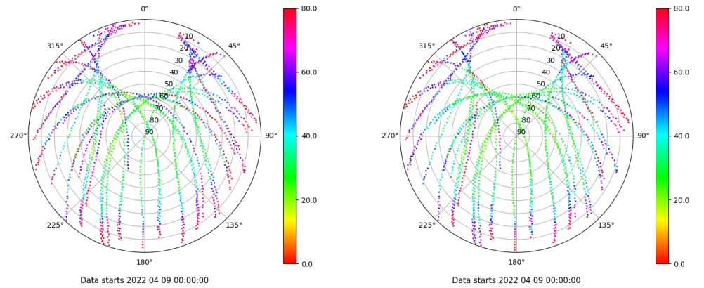
Skyplot for station VIGO. Parameter M1C Data file VIGO00ESP_R_2022099.xtr Skyplot for station VIGO. Parameter M2C Data file VIGO00ESP_R_2022099.xtr
