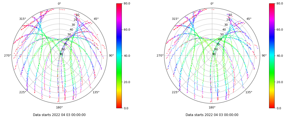
Skyplot for station VIGO. Parameter M1C Data file VIGO00ESP_R_2022093.xtr Skyplot for station VIGO. Parameter M2C Data file VIGO00ESP_R_2022093.xtr
