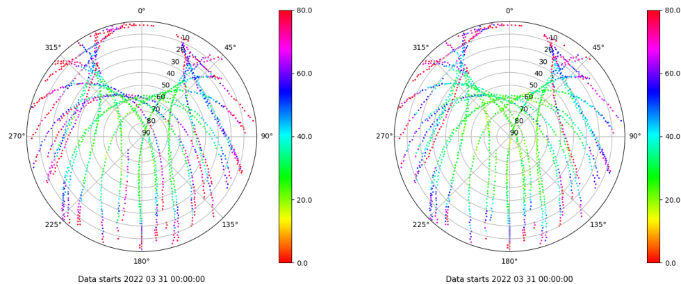
Skyplot for station VIGO. Parameter M1C Data file VIGO00ESP_R_2022090.xtr Skyplot for station VIGO. Parameter M2C Data file VIGO00ESP_R_2022090.xtr
