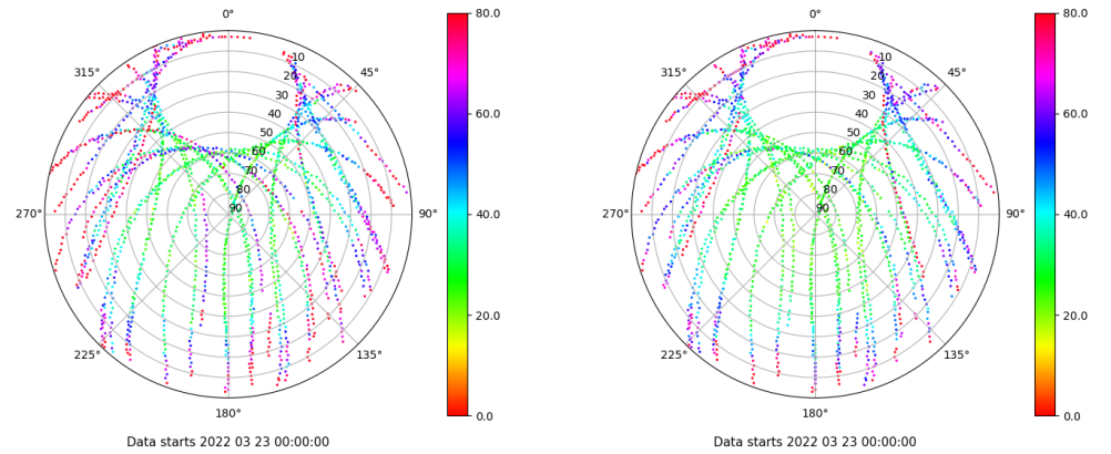
Skyplot for station VIGO. Parameter M1C Data file VIGO00ESP_R_2022082.xtr Skyplot for station VIGO. Parameter M2C Data file VIGO00ESP_R_2022082.xtr
