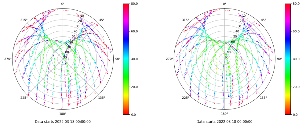
Skyplot for station VIGO. Parameter M1C Data file VIGO00ESP_R_2022077.xtr Skyplot for station VIGO. Parameter M2C Data file VIGO00ESP_R_2022077.xtr
