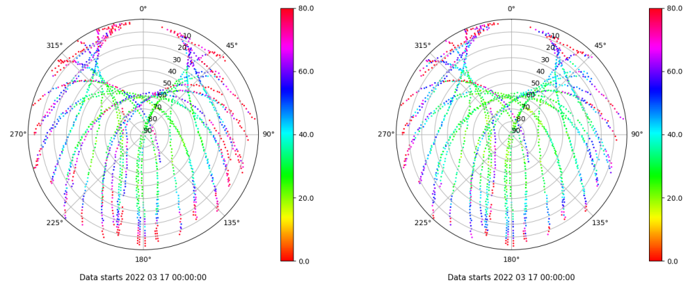
Skyplot for station VIGO. Parameter M1C Data file VIGO00ESP_R_2022076.xtr Skyplot for station VIGO. Parameter M2C Data file VIGO00ESP_R_2022076.xtr
