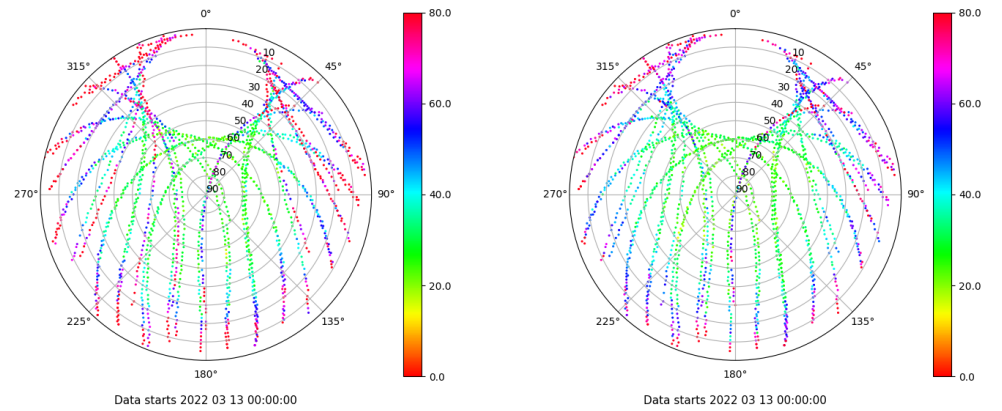
Skyplot for station VIGO. Parameter M1C Data file VIGO00ESP_R_2022072.xtr Skyplot for station VIGO. Parameter M2C Data file VIGO00ESP_R_2022072.xtr
