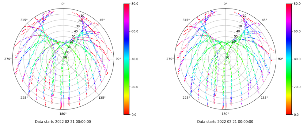
Skyplot for station VIGO. Parameter M1C Data file VIGO00ESP_R_2022052.xtr Skyplot for station VIGO. Parameter M2C Data file VIGO00ESP_R_2022052.xtr
