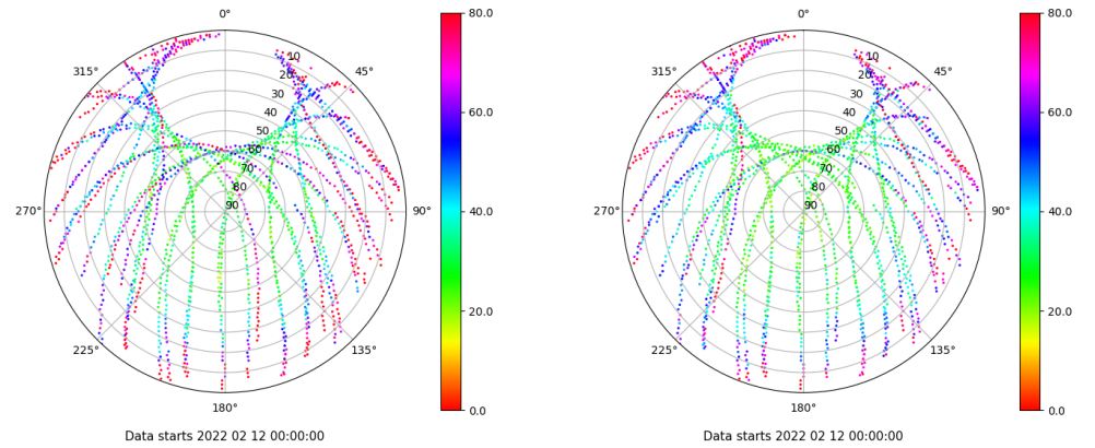
Skyplot for station VIGO. Parameter M1C Data file VIGO00ESP_R_2022043.xtr Skyplot for station VIGO. Parameter M2C Data file VIGO00ESP_R_2022043.xtr
