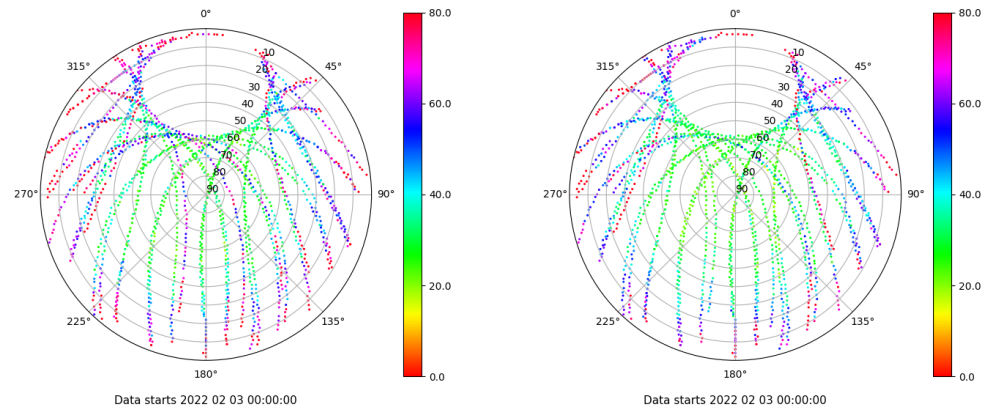
Skyplot for station VIGO. Parameter M1C Data file VIGO00ESP_R_2022034.xtr Skyplot for station VIGO. Parameter M2C Data file VIGO00ESP_R_2022034.xtr
