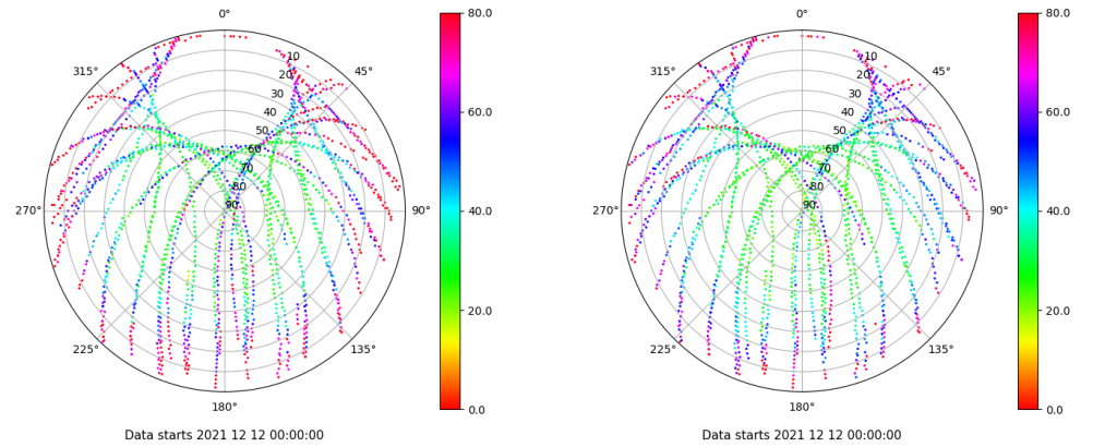
Skyplot for station VIGO. Parameter M1C Data file VIGO00ESP_R_2021346.xtr Skyplot for station VIGO. Parameter M2C Data file VIGO00ESP_R_2021346.xtr
