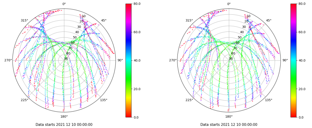
Skyplot for station VIGO. Parameter M1C Data file VIGO00ESP_R_2021344.xtr Skyplot for station VIGO. Parameter M2C Data file VIGO00ESP_R_2021344.xtr
