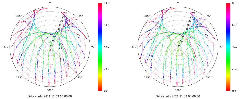
Skyplot for station VIGO. Parameter M1C Data file VIGO00ESP_R_2021307.xtr Skyplot for station VIGO. Parameter M2C Data file VIGO00ESP_R_2021307.xtr
