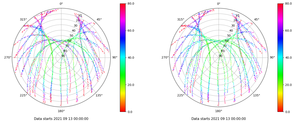
Skyplot for station VIGO. Parameter M1C Data file VIGO00ESP_R_2021256.xtr Skyplot for station VIGO. Parameter M2C Data file VIGO00ESP_R_2021256.xtr
