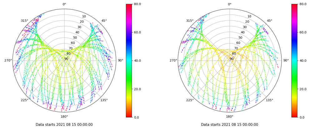
Skyplot for station VIGO. Parameter M1C Data file VIGO00ESP_R_2021227.xtr Skyplot for station VIGO. Parameter M2X Data file VIGO00ESP_R_2021227.xtr
