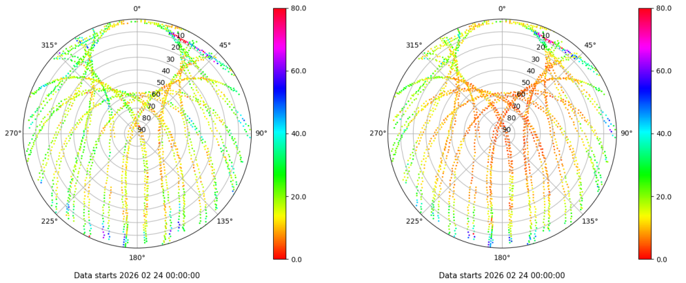
Skyplot for station VALA. Parameter M1C Data file VALA00ESP_R_2026055.xtr Skyplot for station VALA. Parameter M2C Data file VALA00ESP_R_2026055.xtr
