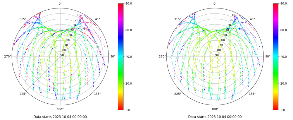
Skyplot for station ULP2. Parameter M1C Data file ULP200ESP_R_2023277.xtr Skyplot for station ULP2. Parameter M2C Data file ULP200ESP_R_2023277.xtr
