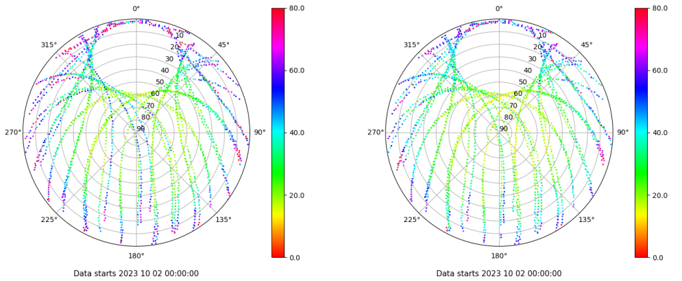
Skyplot for station TUD1. Parameter M1C Data file TUD100ESP_R_2023275.xtr Skyplot for station TUD1. Parameter M2C Data file TUD100ESP_R_2023275.xtr
