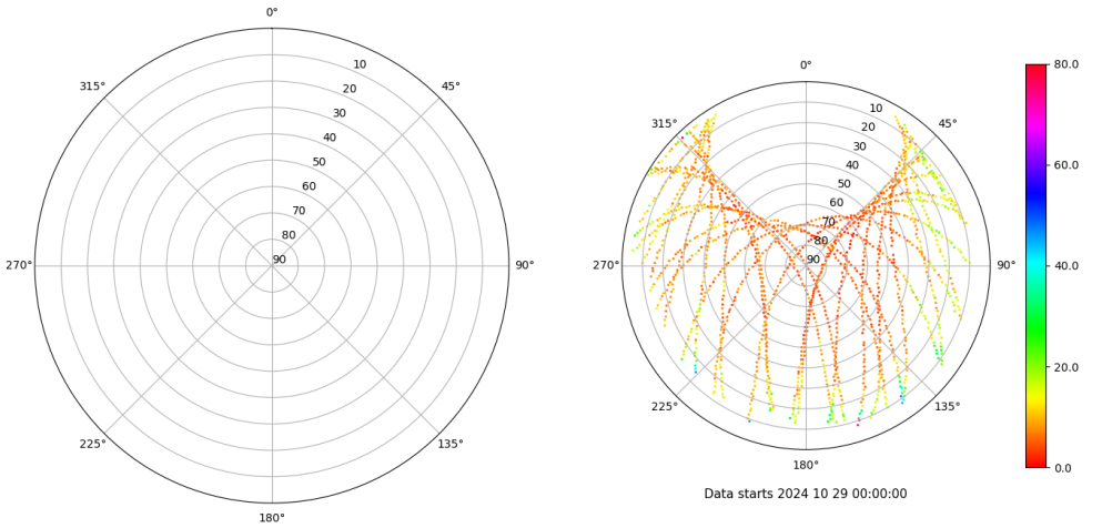
Skyplot for station TRAU. Parameter M1C Data file TRAU00ESP_R_2024303.xtr Skyplot for station TRAU. Parameter M2S Data file TRAU00ESP_R_2024303.xtr
