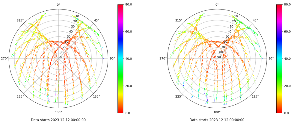
Skyplot for station TARR. Parameter M1C Data file TARR00ESP_R_2023346.xtr Skyplot for station TARR. Parameter M2P Data file TARR00ESP_R_2023346.xtr
