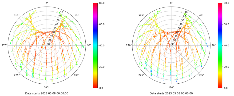
Skyplot for station TARR. Parameter M1C Data file TARR00ESP_R_2023128.xtr Skyplot for station TARR. Parameter M2P Data file TARR00ESP_R_2023128.xtr
