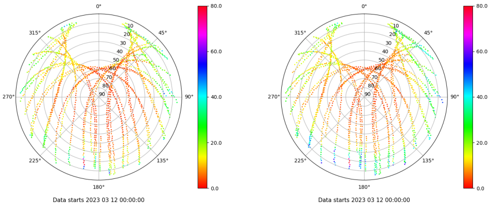
Skyplot for station TARR. Parameter M1C Data file TARR00ESP_R_2023071.xtr Skyplot for station TARR. Parameter M2P Data file TARR00ESP_R_2023071.xtr
