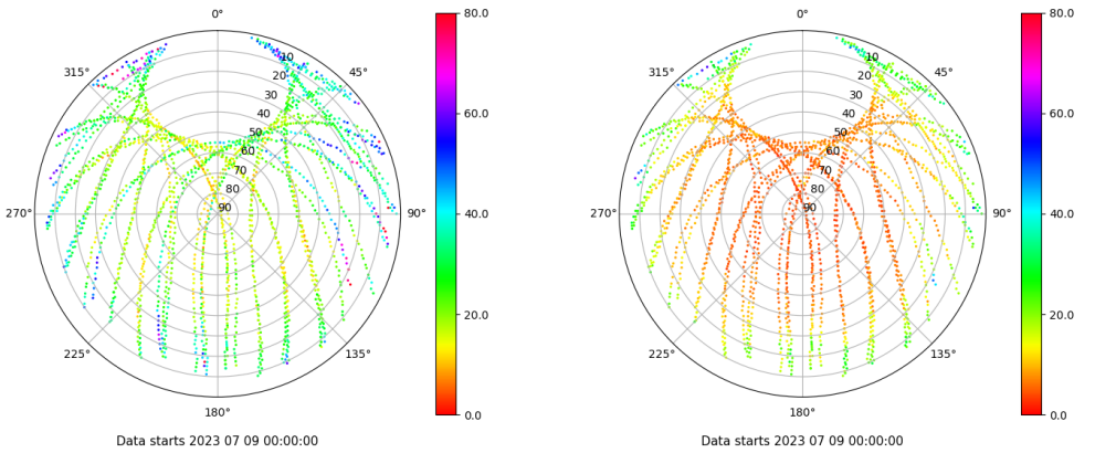
Skyplot for station SPAB. Parameter M1C Data file SPAB00ESP_R_2023190.xtr Skyplot for station SPAB. Parameter M2P Data file SPAB00ESP_R_2023190.xtr
