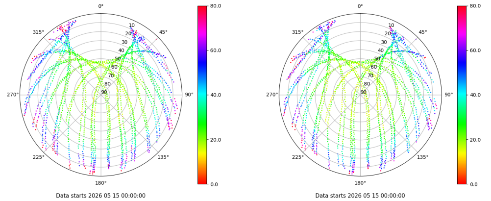
Skyplot for station SEV1. Parameter M1C Data file SEV100ESP_R_2026135.xtr Skyplot for station SEV1. Parameter M2C Data file SEV100ESP_R_2026135.xtr
