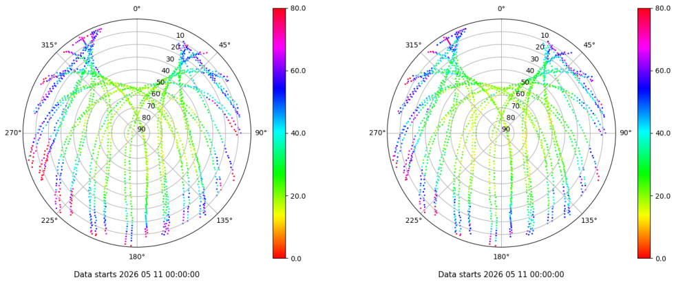
Skyplot for station SEV1. Parameter M1C Data file SEV100ESP_R_2026131.xtr Skyplot for station SEV1. Parameter M2C Data file SEV100ESP_R_2026131.xtr
