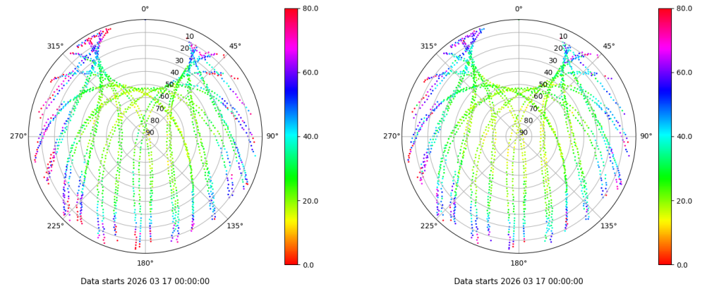
Skyplot for station SEV1. Parameter M1C Data file SEV100ESP_R_2026076.xtr Skyplot for station SEV1. Parameter M2C Data file SEV100ESP_R_2026076.xtr
