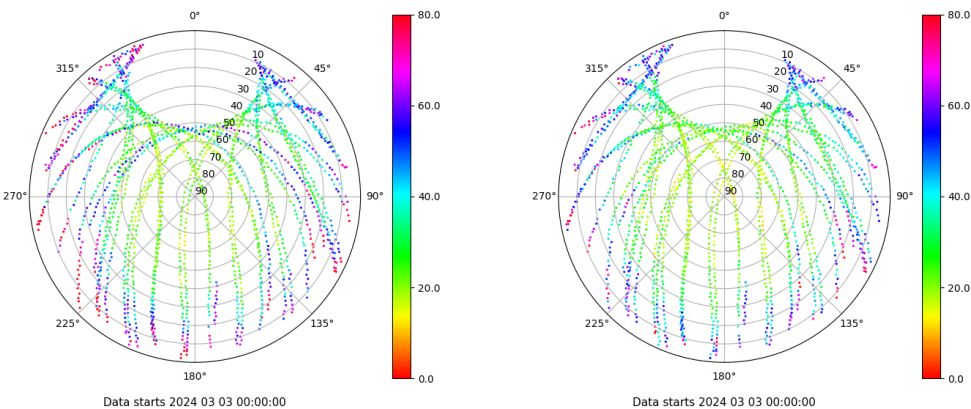
Skyplot for station SEV1. Parameter M1C Data file SEV100ESP_R_2024063.xtr Skyplot for station SEV1. Parameter M2C Data file SEV100ESP_R_2024063.xtr
