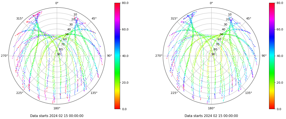
Skyplot for station SEV1. Parameter M1C Data file SEV100ESP_R_2024046.xtr Skyplot for station SEV1. Parameter M2C Data file SEV100ESP_R_2024046.xtr
