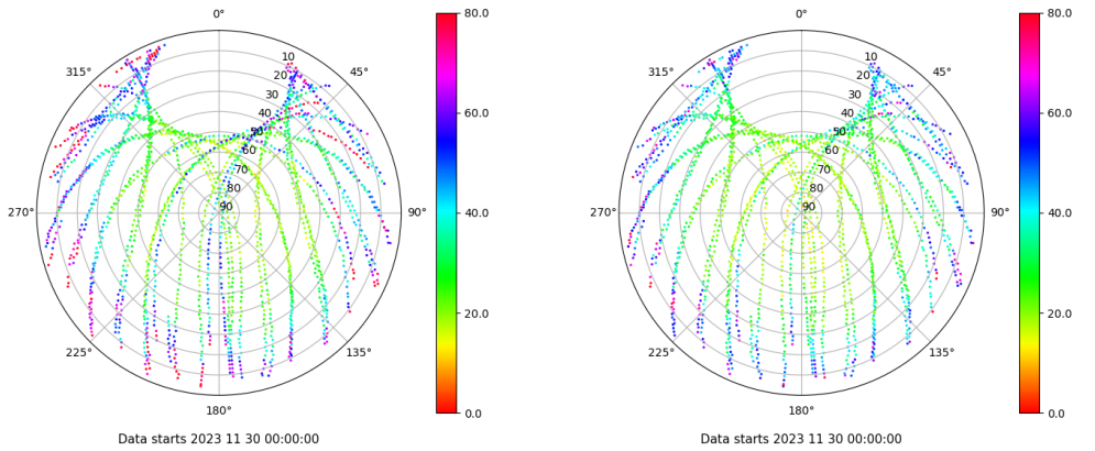
Skyplot for station SEV1. Parameter M1C Data file SEV100ESP_R_2023334.xtr Skyplot for station SEV1. Parameter M2C Data file SEV100ESP_R_2023334.xtr
