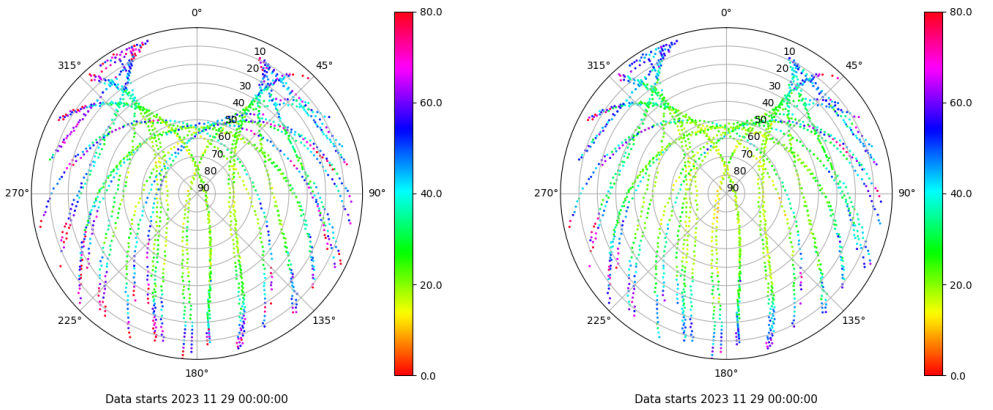
Skyplot for station SEV1. Parameter M1C Data file SEV100ESP_R_2023333.xtr Skyplot for station SEV1. Parameter M2C Data file SEV100ESP_R_2023333.xtr
