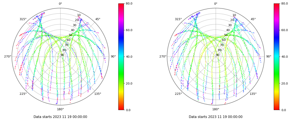
Skyplot for station SEV1. Parameter M1C Data file SEV100ESP_R_2023323.xtr Skyplot for station SEV1. Parameter M2C Data file SEV100ESP_R_2023323.xtr
