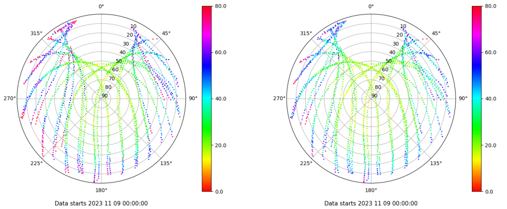
Skyplot for station SEV1. Parameter M1C Data file SEV100ESP_R_2023313.xtr Skyplot for station SEV1. Parameter M2C Data file SEV100ESP_R_2023313.xtr
