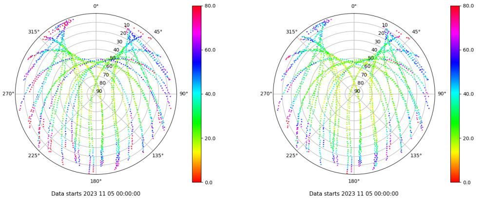
Skyplot for station SEV1. Parameter M1C Data file SEV100ESP_R_2023309.xtr Skyplot for station SEV1. Parameter M2C Data file SEV100ESP_R_2023309.xtr
