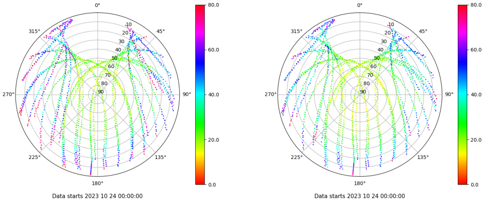
Skyplot for station SEV1. Parameter M1C Data file SEV100ESP_R_2023297.xtr Skyplot for station SEV1. Parameter M2C Data file SEV100ESP_R_2023297.xtr
