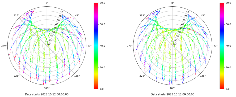
Skyplot for station SEV1. Parameter M1C Data file SEV100ESP_R_2023285.xtr Skyplot for station SEV1. Parameter M2C Data file SEV100ESP_R_2023285.xtr
