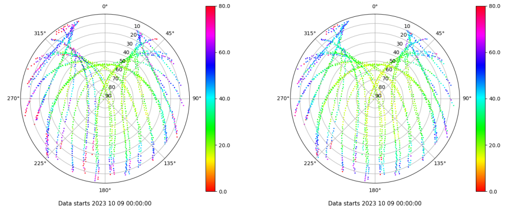
Skyplot for station SEV1. Parameter M1C Data file SEV100ESP_R_2023282.xtr Skyplot for station SEV1. Parameter M2C Data file SEV100ESP_R_2023282.xtr
