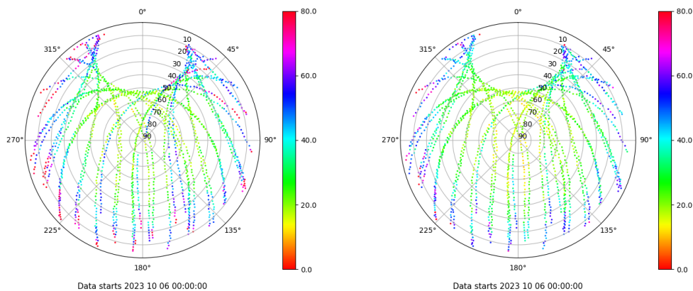
Skyplot for station SEV1. Parameter M1C Data file SEV100ESP_R_2023279.xtr Skyplot for station SEV1. Parameter M2C Data file SEV100ESP_R_2023279.xtr
