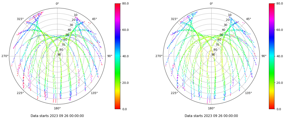
Skyplot for station SEV1. Parameter M1C Data file SEV100ESP_R_2023269.xtr Skyplot for station SEV1. Parameter M2C Data file SEV100ESP_R_2023269.xtr
