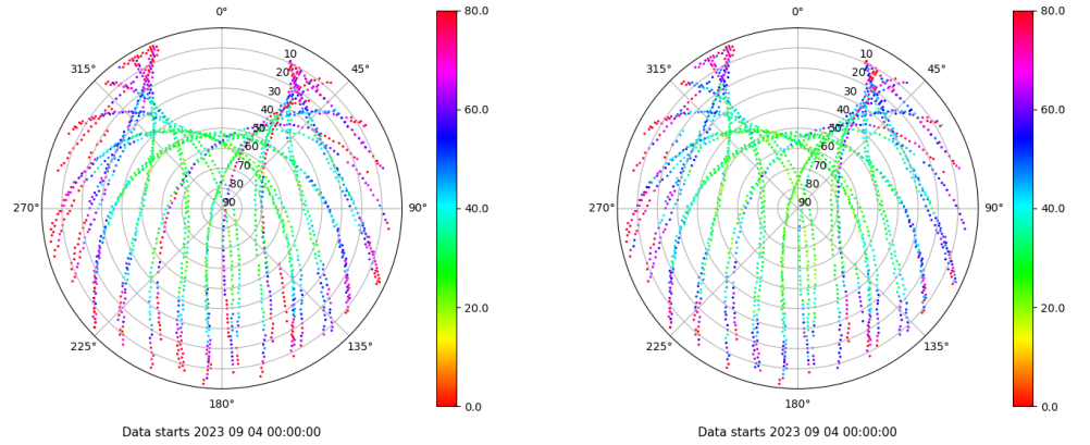
Skyplot for station SEV1. Parameter M1C Data file SEV100ESP_R_2023247.xtr Skyplot for station SEV1. Parameter M2C Data file SEV100ESP_R_2023247.xtr
