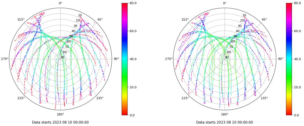
Skyplot for station SEV1. Parameter M1C Data file SEV100ESP_R_2023222.xtr Skyplot for station SEV1. Parameter M2C Data file SEV100ESP_R_2023222.xtr
