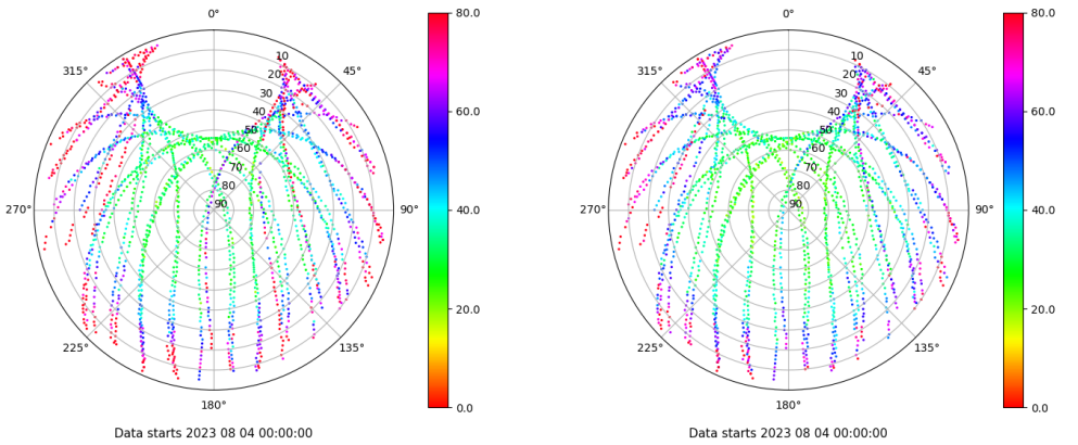
Skyplot for station SEV1. Parameter M1C Data file SEV100ESP_R_2023216.xtr Skyplot for station SEV1. Parameter M2C Data file SEV100ESP_R_2023216.xtr
