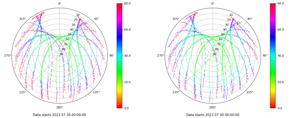
Skyplot for station SEV1. Parameter M1C Data file SEV100ESP_R_2023211.xtr Skyplot for station SEV1. Parameter M2C Data file SEV100ESP_R_2023211.xtr
