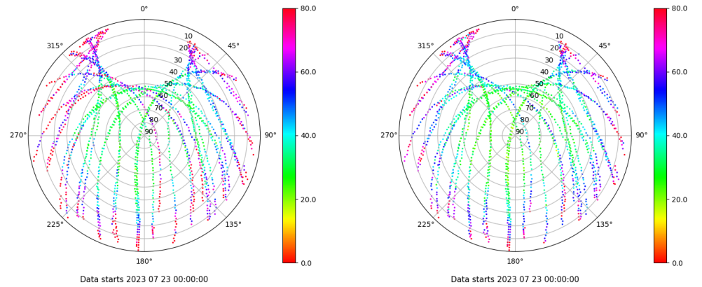
Skyplot for station SEV1. Parameter M1C Data file SEV100ESP_R_2023204.xtr Skyplot for station SEV1. Parameter M2C Data file SEV100ESP_R_2023204.xtr
