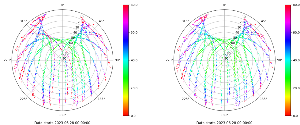
Skyplot for station SEV1. Parameter M1C Data file SEV100ESP_R_2023179.xtr Skyplot for station SEV1. Parameter M2C Data file SEV100ESP_R_2023179.xtr
