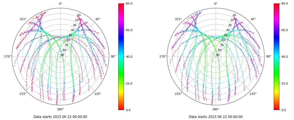
Skyplot for station SEV1. Parameter M1C Data file SEV100ESP_R_2023173.xtr Skyplot for station SEV1. Parameter M2C Data file SEV100ESP_R_2023173.xtr
