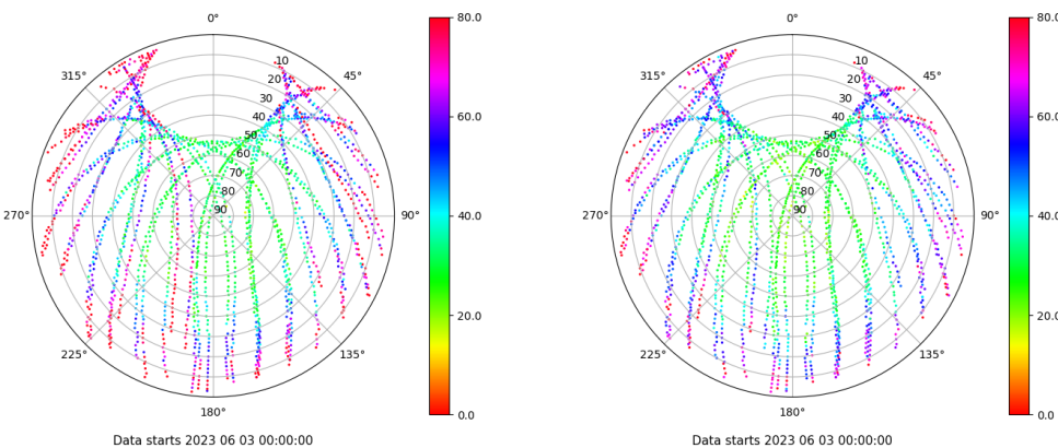
Skyplot for station SEV1. Parameter M1C Data file SEV100ESP_R_2023154.xtr Skyplot for station SEV1. Parameter M2C Data file SEV100ESP_R_2023154.xtr
