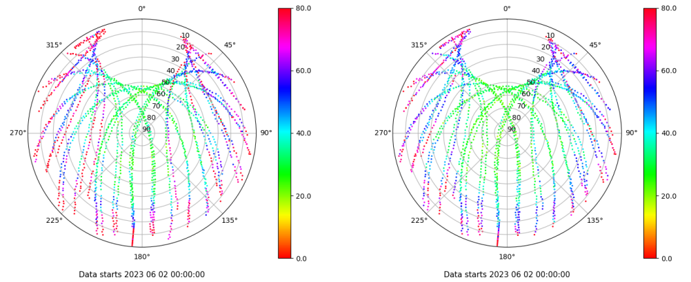
Skyplot for station SEV1. Parameter M1C Data file SEV100ESP_R_2023153.xtr Skyplot for station SEV1. Parameter M2C Data file SEV100ESP_R_2023153.xtr
