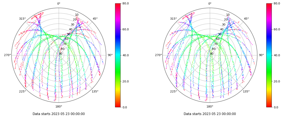
Skyplot for station SEV1. Parameter M1C Data file SEV100ESP_R_2023143.xtr Skyplot for station SEV1. Parameter M2C Data file SEV100ESP_R_2023143.xtr
